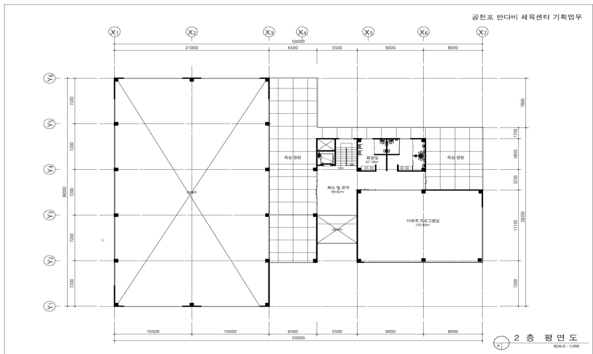
【설 명】 2층 평면도
