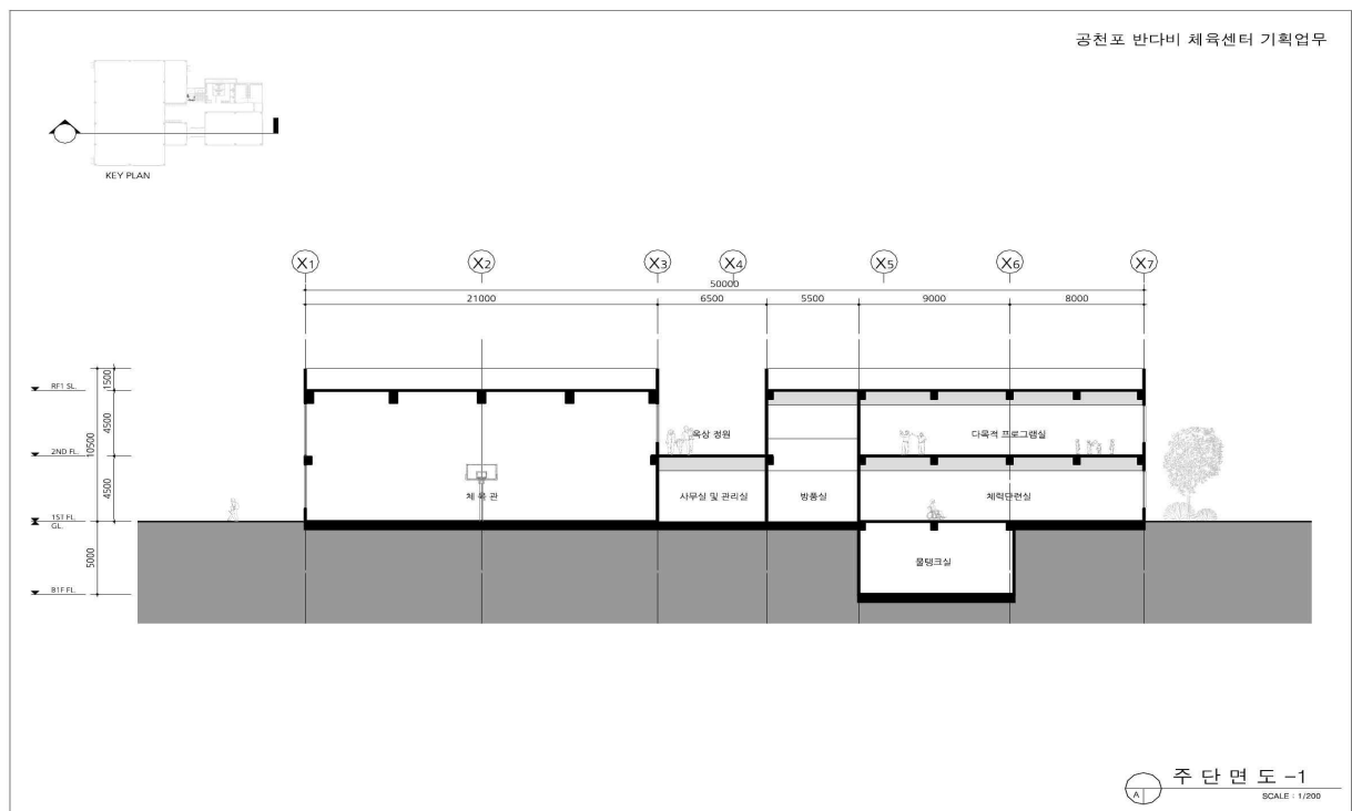
【설 명】 단 면 도
